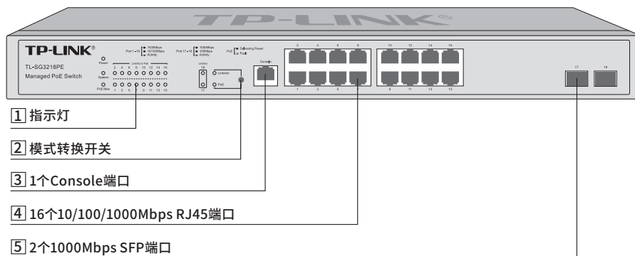
图1-9 TL-SG3218PE前面板示意图
