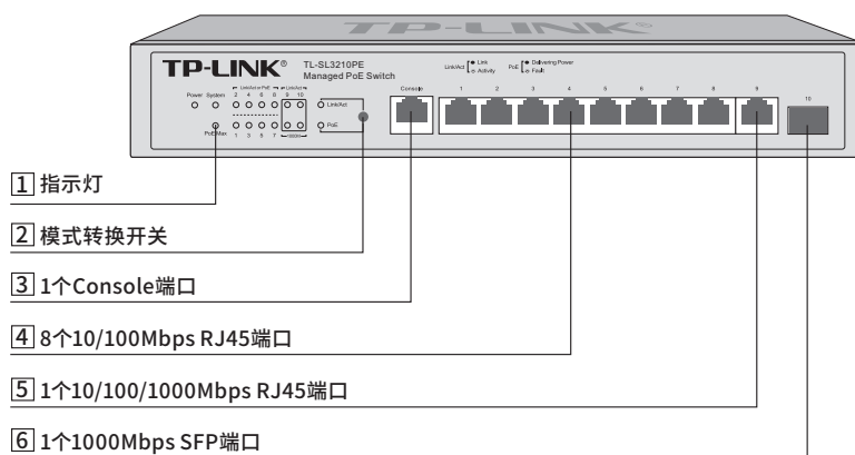
图1-22 TL-SL3210PE前面板示意图
