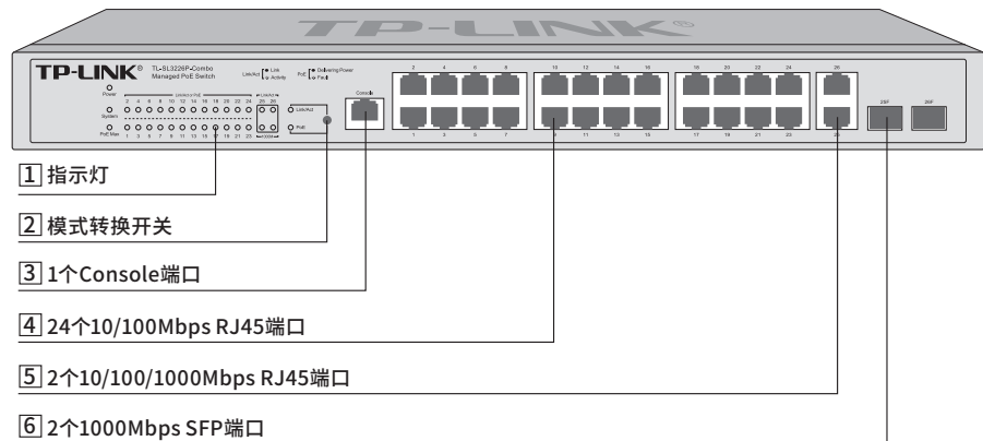
图1-20 TL-SL3226P-Combo前面板示意图
