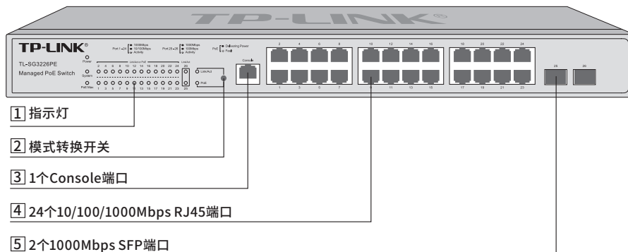
图1-7 TL-SG3226PE前面板示意图
