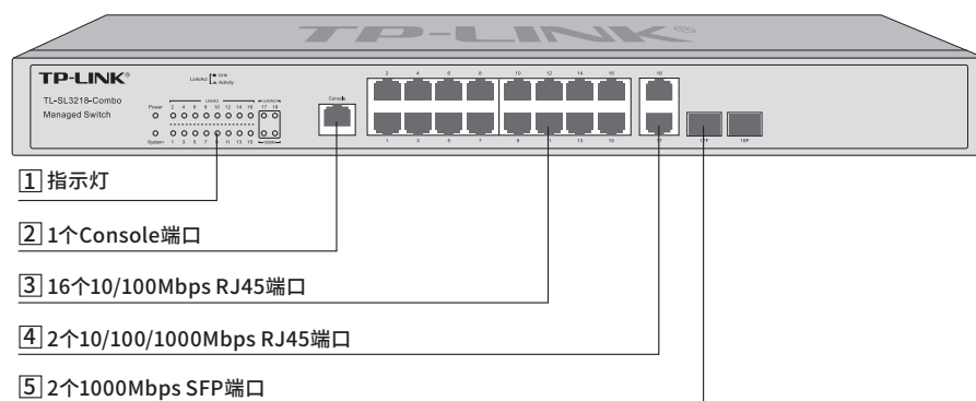
图1-15 TL-SL3218-Combo前面板示意图
