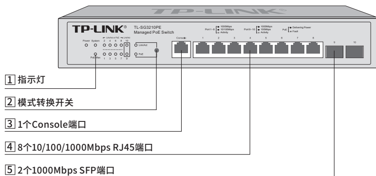
图1-10 TL-SG3210PE前面板示意图
