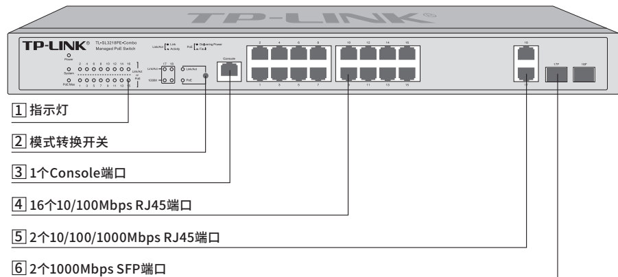
图1-21 TL-SL3218PE-Combo前面板示意图
