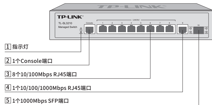
图1-17 TL-SL3210前面板示意图
