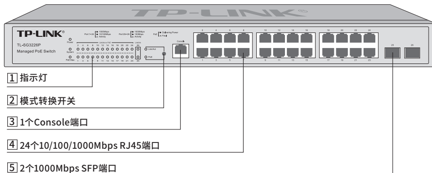
图1-8 TL-SG3226P前面板示意图
