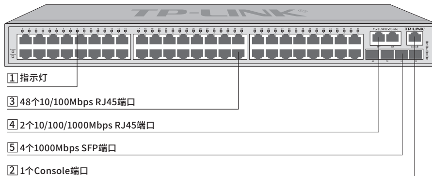
图1-11 TL-SL3452-Combo前面板示意图
