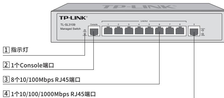
图1-18 TL-SL3109前面板示意图
