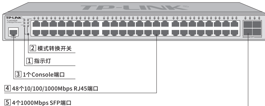
图1-6 TL-SG3452P前面板示意图
