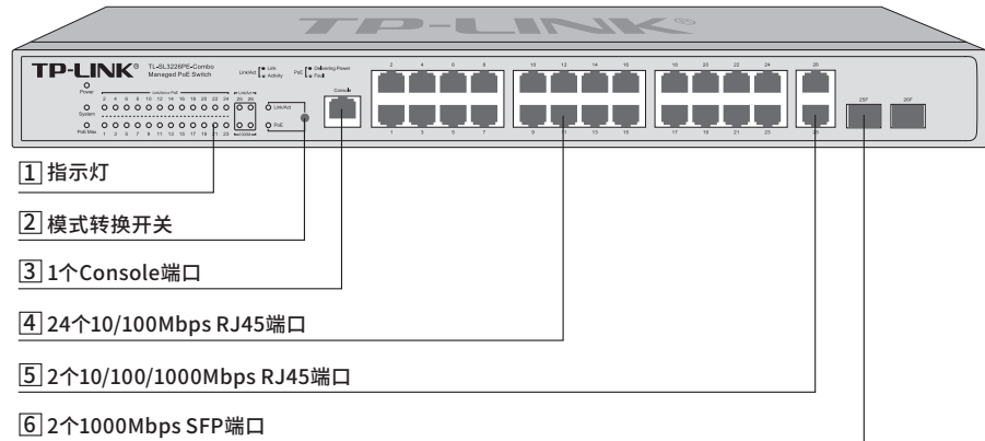
图1-19 TL-SL3226PE-Combo前面板示意图
