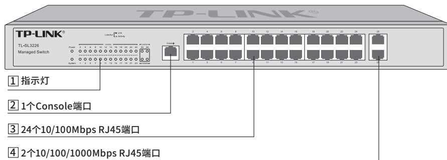
图1-14 TL-SL3226前面板示意图
