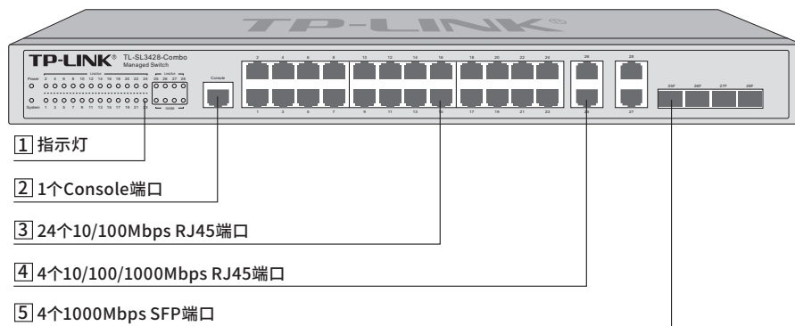
图1-12 TL-SL3428-Combo前面板示意图
