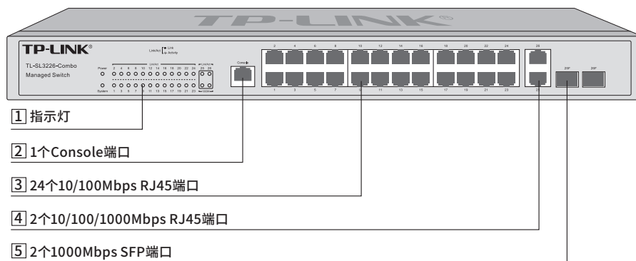
图1-13 TL-SL3226-Combo前面板示意图
