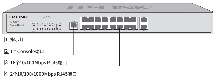
图1-16 TL-SL3218前面板示意图
